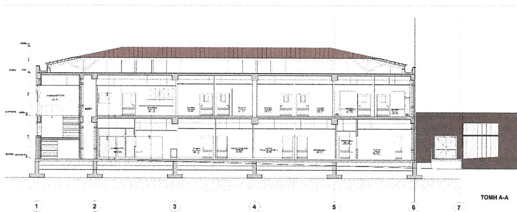
ΤΟΜΗ Α-Α
